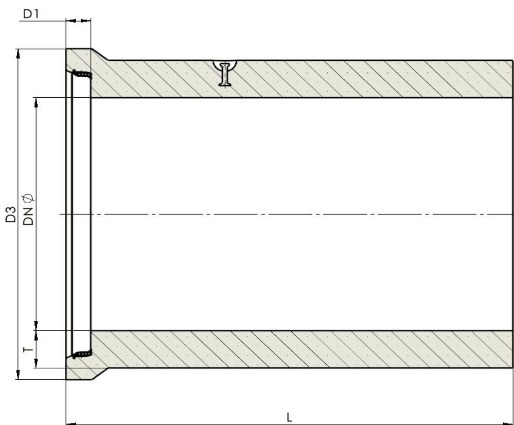
HRDLO - VÝTOK
