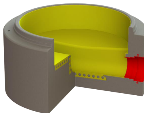
DETAIL ŠACHTOVÉHO DNA DN 1000/500
